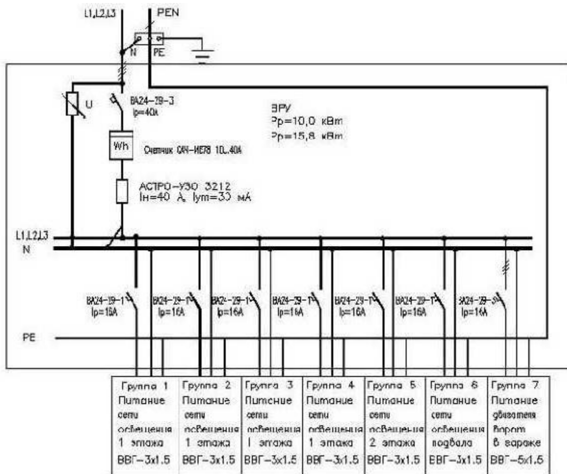
Рисунок 1– Однолинейная схема трансформаторной подстанции.
